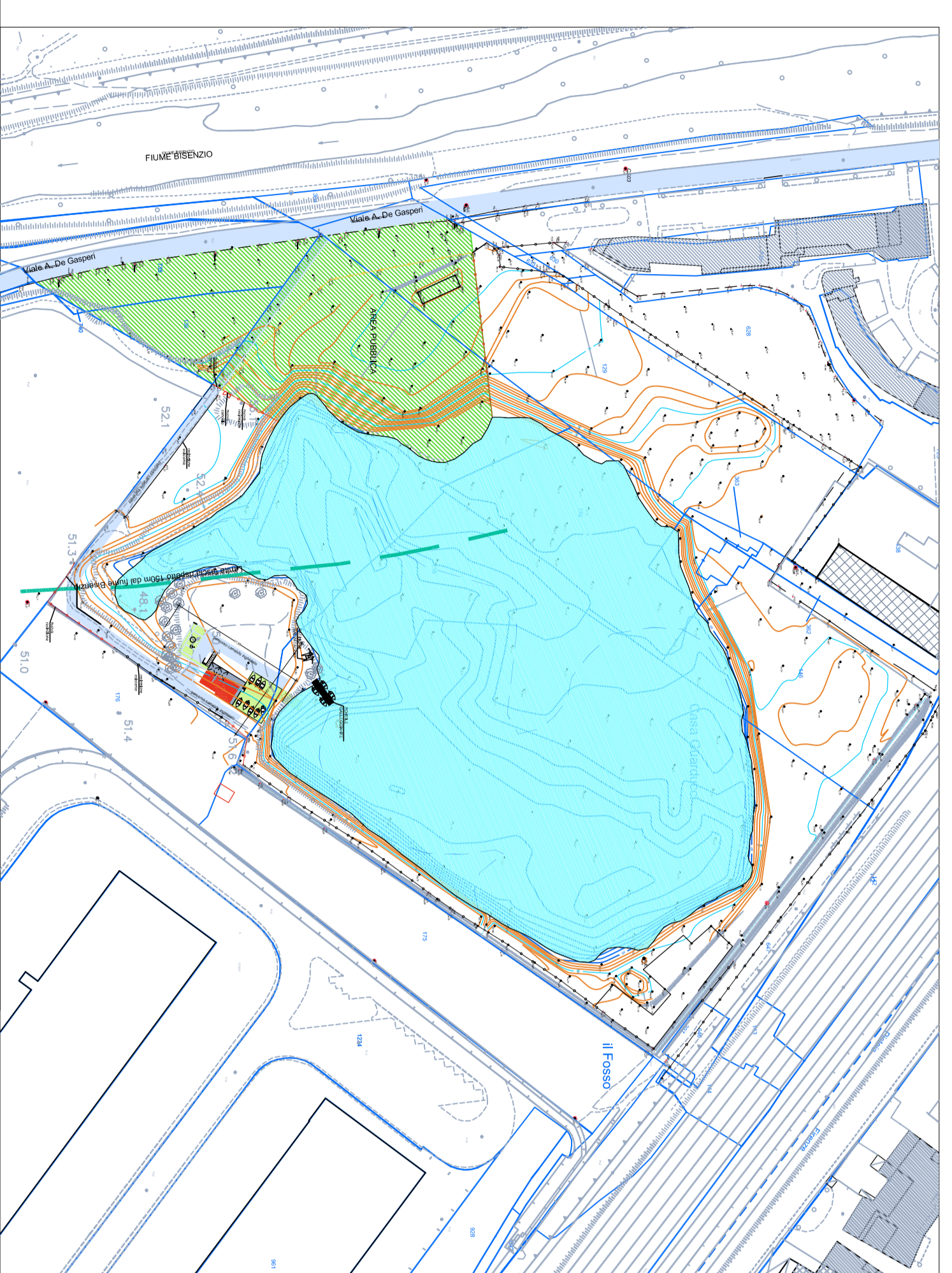
PLANIMETRIA GENERALE - SCALA 1:2000
